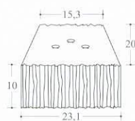
NORMÁLKŐ 50 db/m 2
