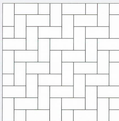
Térköszükséglet 1 m 2 : 10x20 cm-es téglá kb. 50 db
