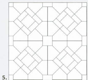
5. Térköszükséglet kb. 0,58 m 2 : 10x20 cm-es téglák 6 db 20x20 cm-es kocka 2 db kezdőkő 8 db
