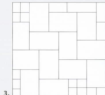
3. Térköszükséglet 1 m 2 : 20x30 cm-es nagytégla 17 db szegély: 10x10 cm-es téglák kb. 9 db/fm
