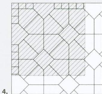
4. Térköszükséglet kb. 0,92 m 2 : 20x20 cm-es kocka 4 db kezdőkő 16 db
